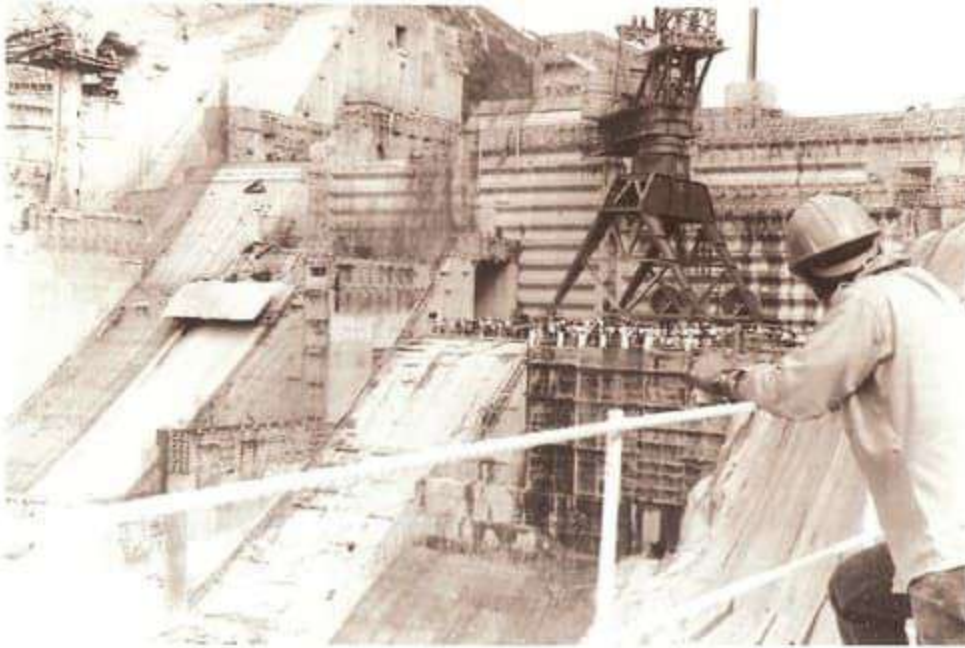
1. Presa y Central Hidroeléctrica "Luis Donaldo Colosio Murrieta". 29 de mayo de 2015.
